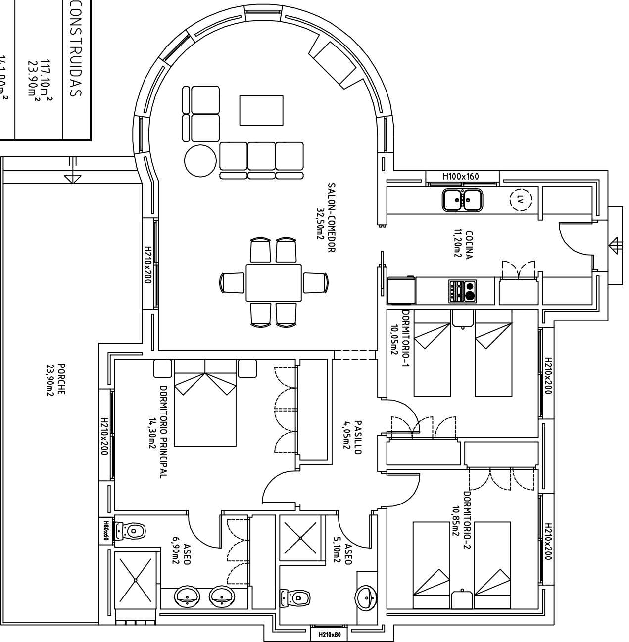
PLANTA BAJA
